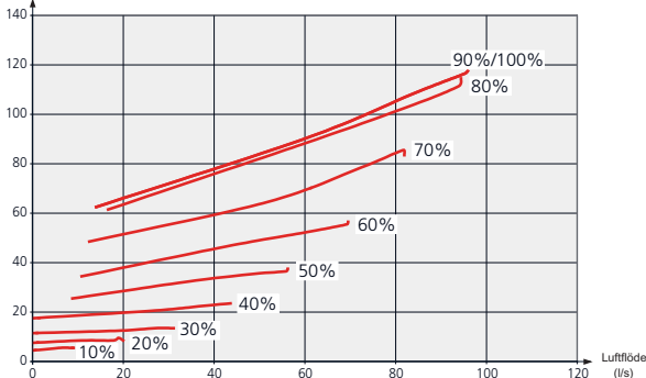
Effekt likströmsfläkt
