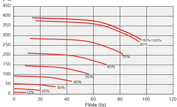
Fläktdiagram F370
