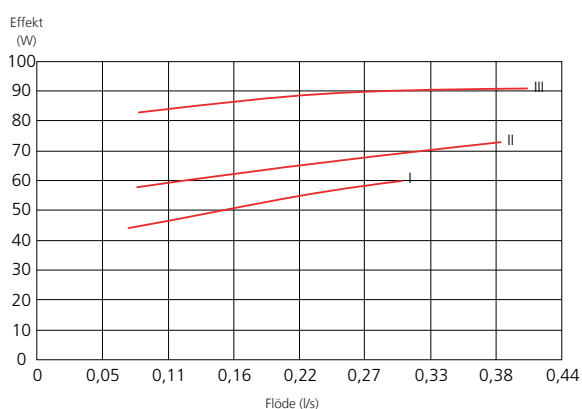
Effekt cirkulationspump
