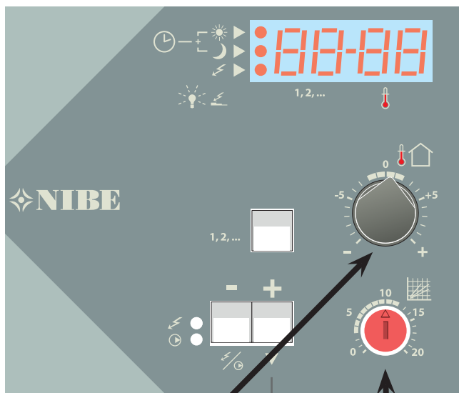
Förskjutning värmekurva
