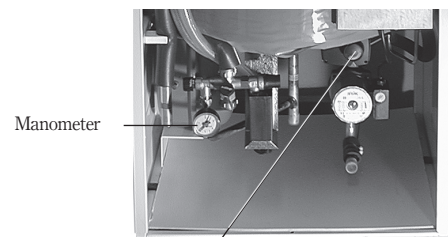
Shuntventil
