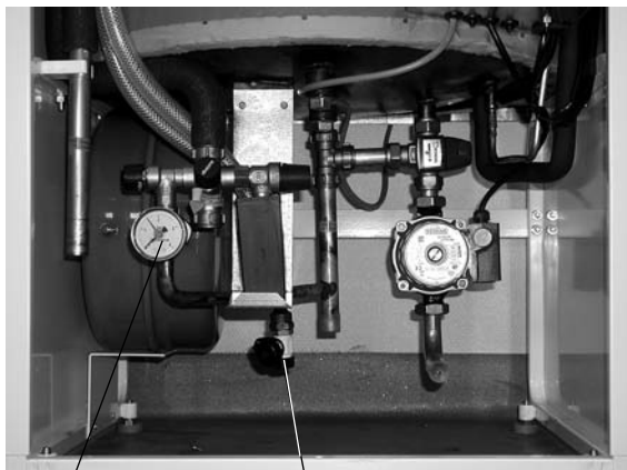
1. Manometer
