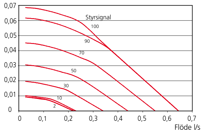
Tryckfallsdiagram VB-pump
