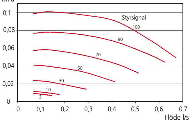
Tryckfallsdiagram KB-pump
